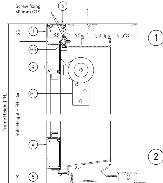
Open Inward Hinged Door Option
