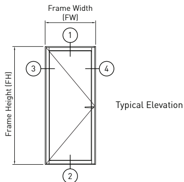
Open Inward Hinged Door Option
